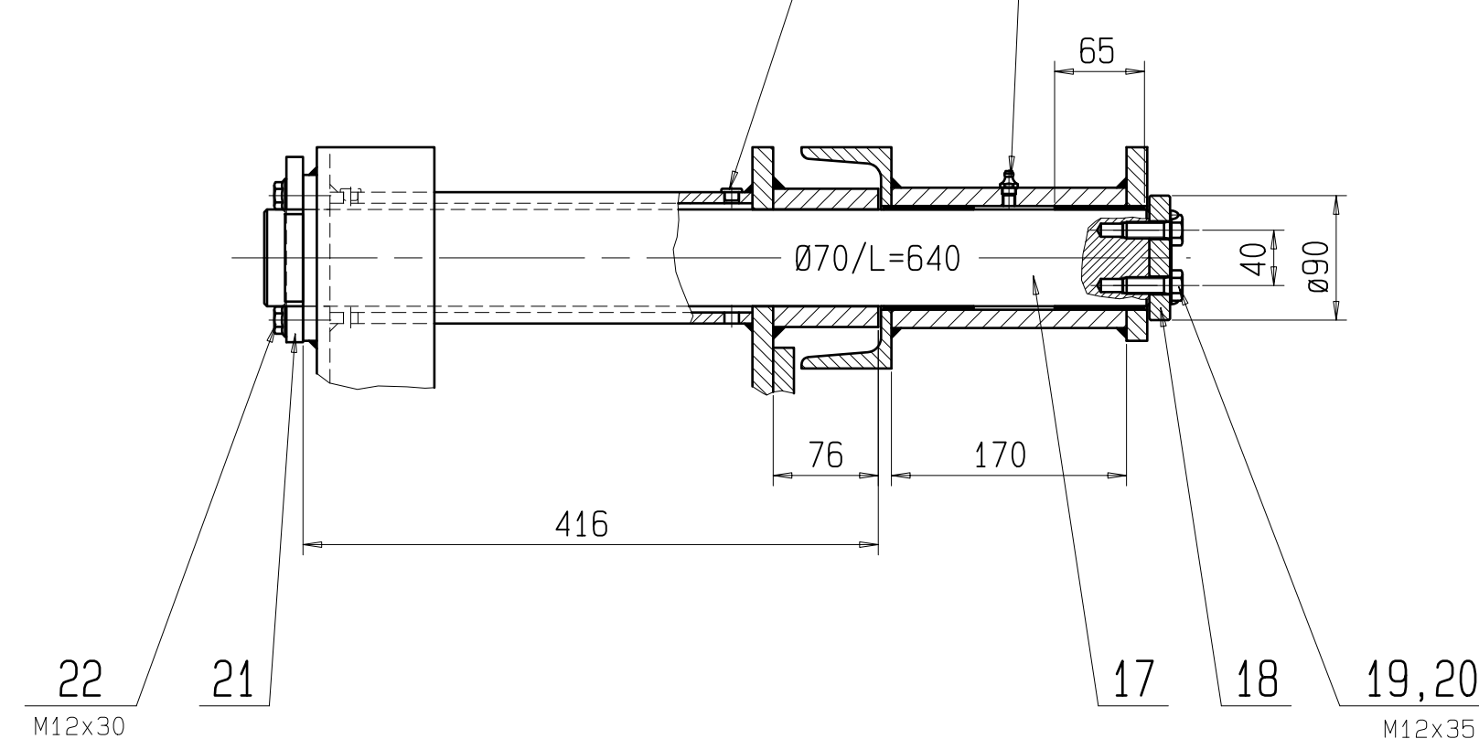
SECTION C-C Maßstab/Scale 1:5
