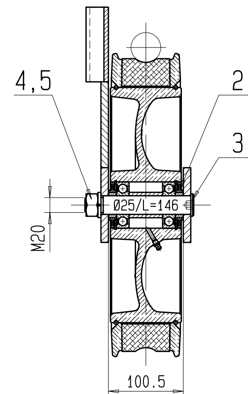
Schnitt A-A M 1:5
