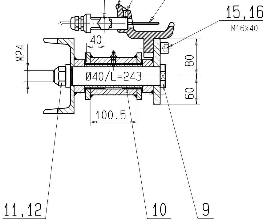
SECTION B-B Maßstab/Scale 1:5
